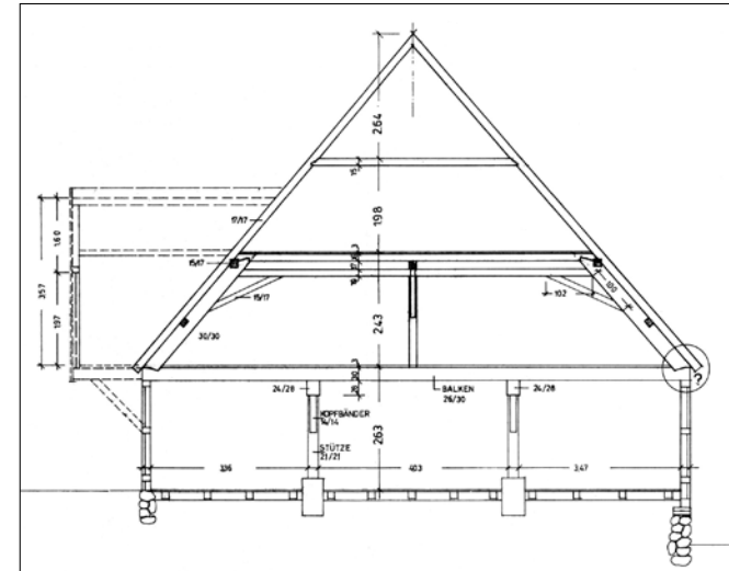
Abb. 4: Schnitt der Moissburger Mühle
