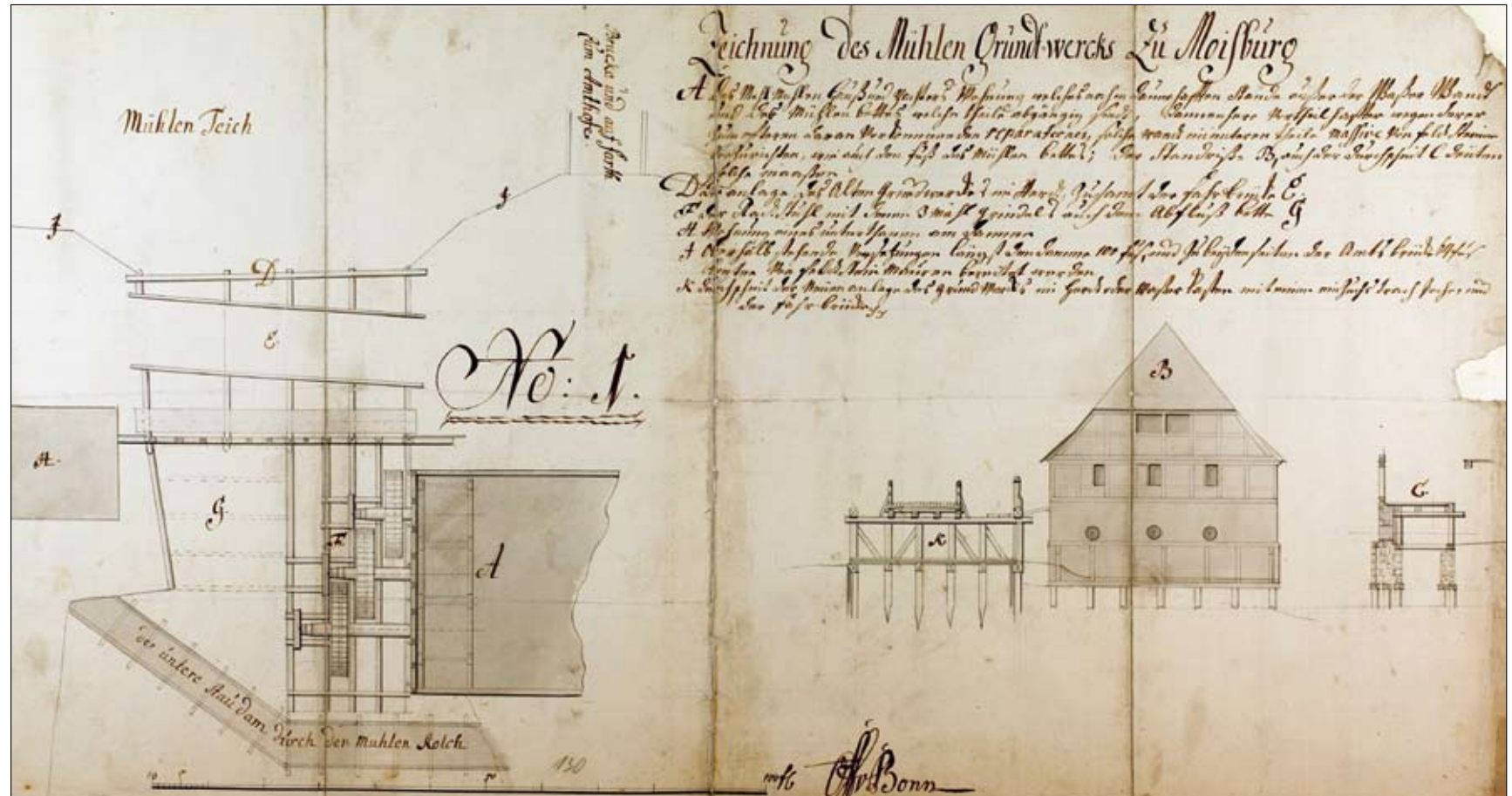
Abb. 7: Zeichnung des Mühlengrundwerks Foto HStAH Karten Nr. 33g Moisburg
